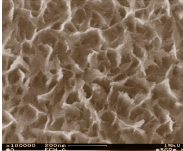
Exemple de nouvelles propriétés par nanostructuration : en s'inspirant de la feuille de nénuphar, une surface d'alumine est rendue hydrophobe par nanostructuration [document Saint-Gobain].
