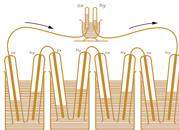
Pile à combustible (Stack of fuel) construite par Sir William Robert GROVE en 1839.
