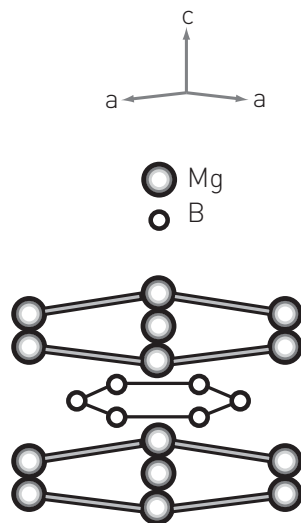
Structure cristalline de MgB 2 (a = 3,086 Å, c = 3,524 Å) d'après : M. Jones et R. Marsh, J. Am. Chem. Soc. 76, 1434-1436, 1954 et J. Nagamatsu, N. Nakagawa, T. Muranaka, Y. Zenitani & J. Akimitsu, Nature 410, 63-64, 2001.
