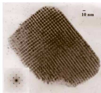
Super-réseau de nanoparticules de fer. Les particules individuelles sont cubiques et toutes orientées dans la même direction.
